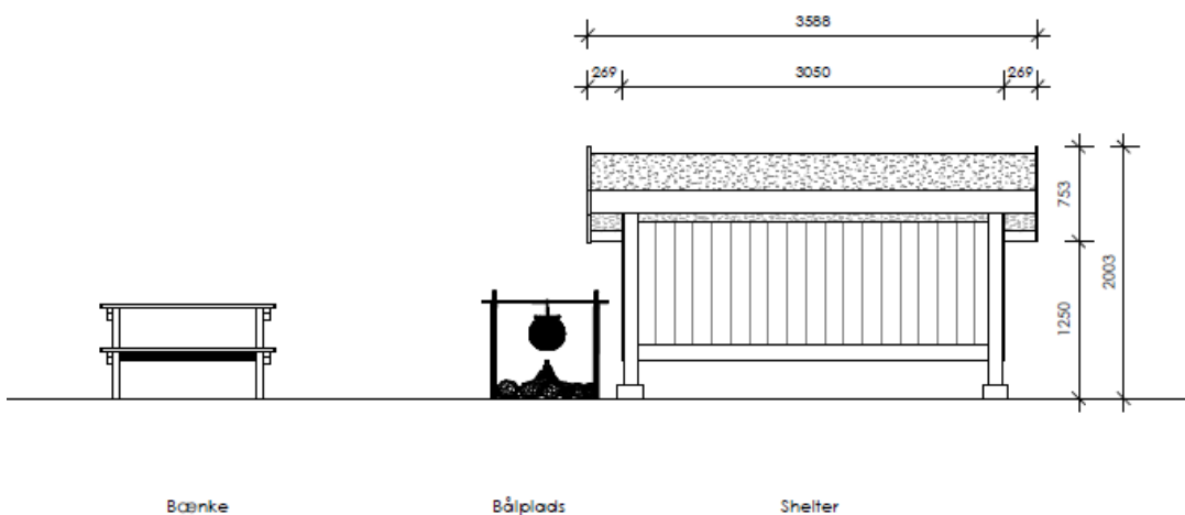
Situationsplan af shelterpladsen. Eksempel af facade.
