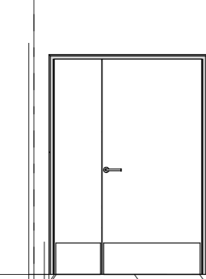
IGP.031 1 : 50
