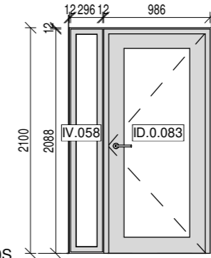
IGP.035 1 : 50
