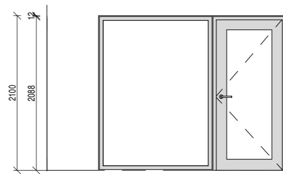
IGP.045 1 : 50
