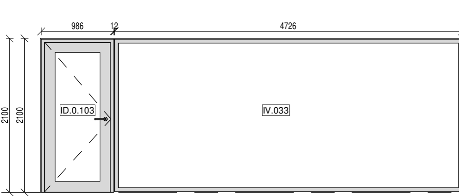
IGP.043 1 : 50
