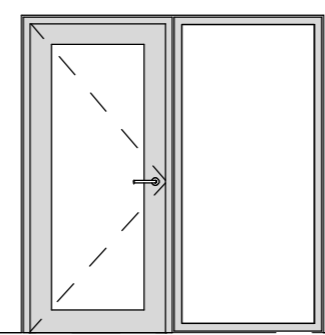
IGP.039 1 : 50
