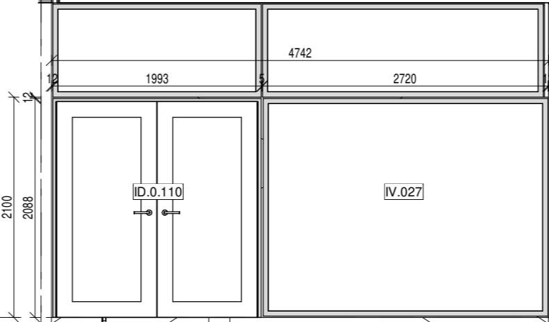
IGP.033 1 : 50
