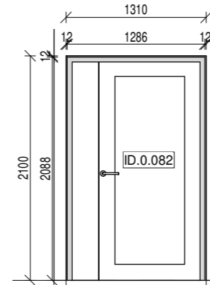
IGP.034 1 : 50
