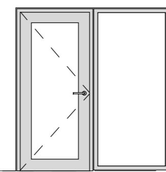
IGP.041 1 : 50
