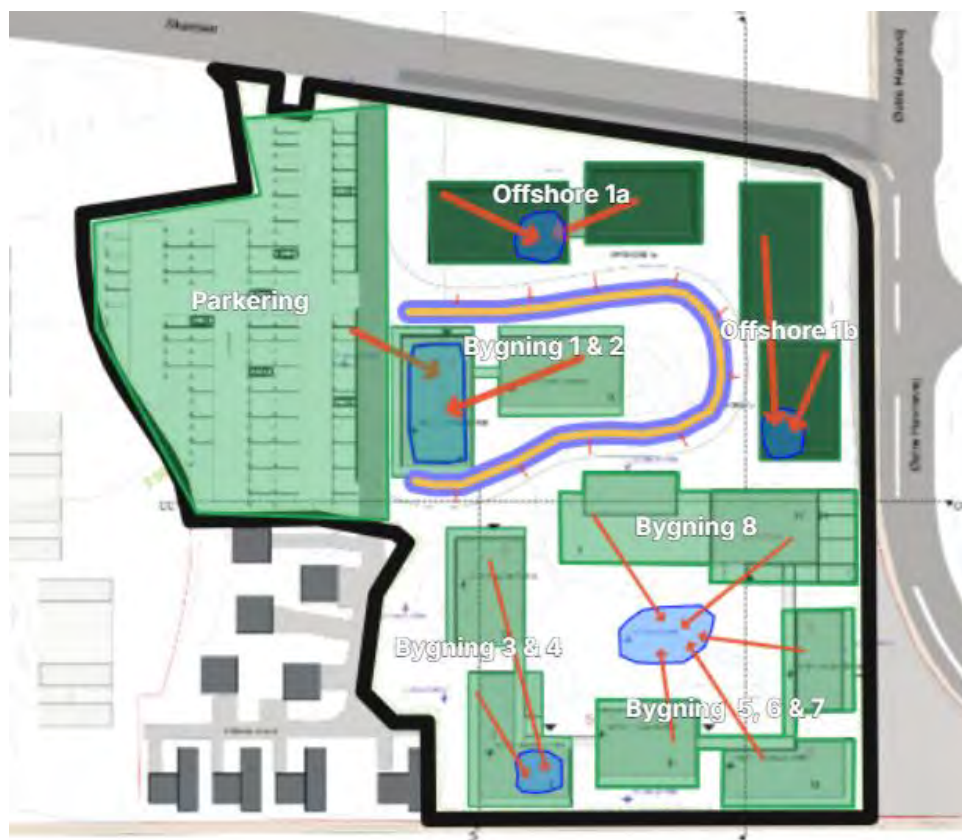
Figur 9.7: Forslag til placering af regnbede markeret med blå og grøft markeret med gul.
